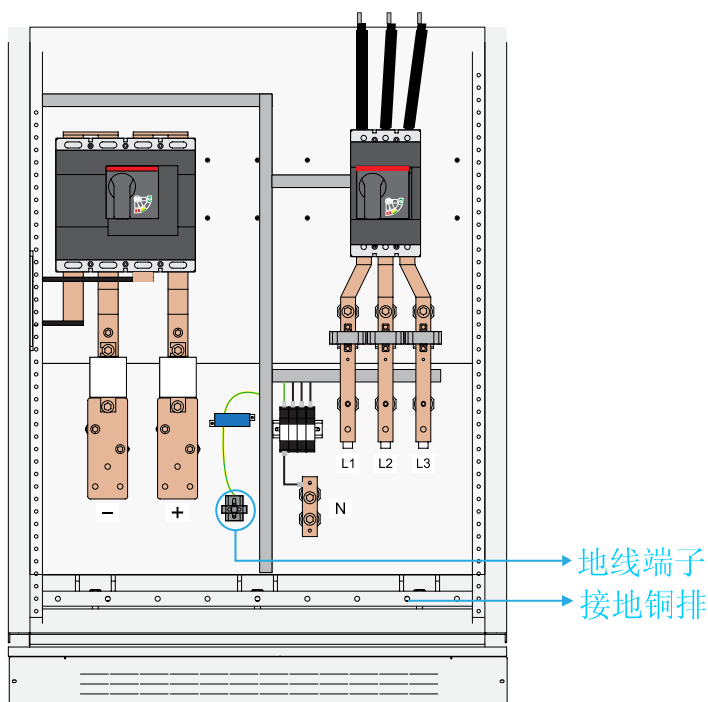
图8-8 接地铜排示意图
