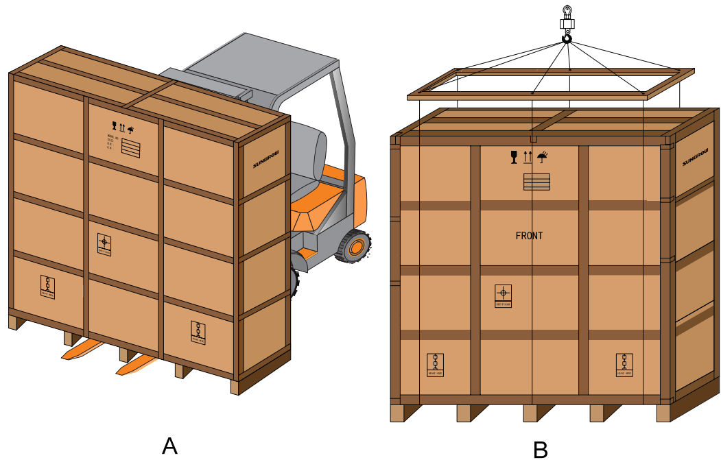
图7-1 带包装逆变器运输
