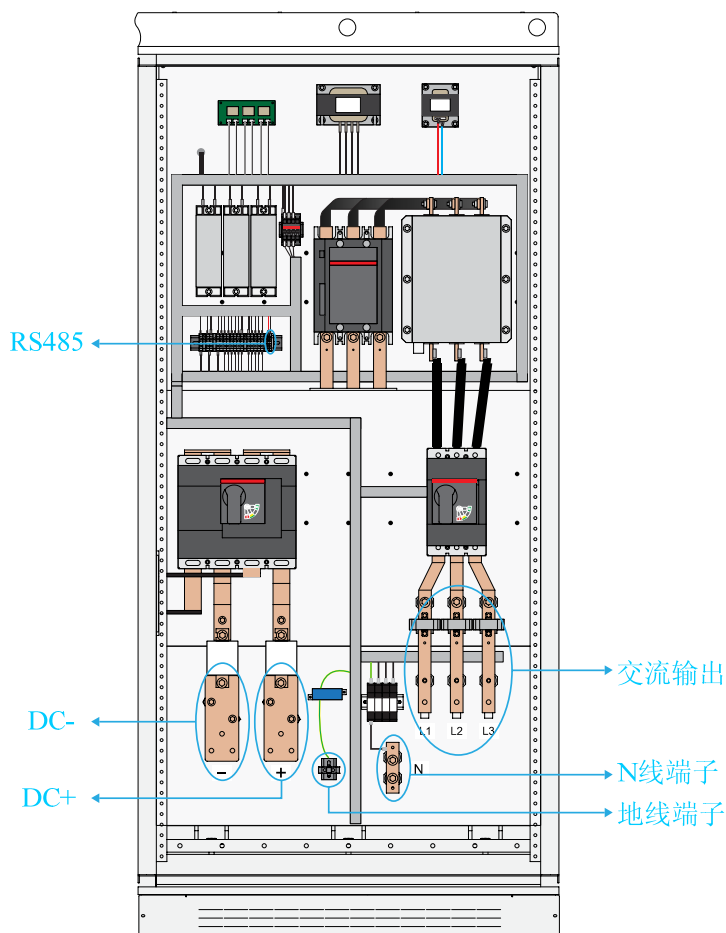
图4-6 接线端子示意图
