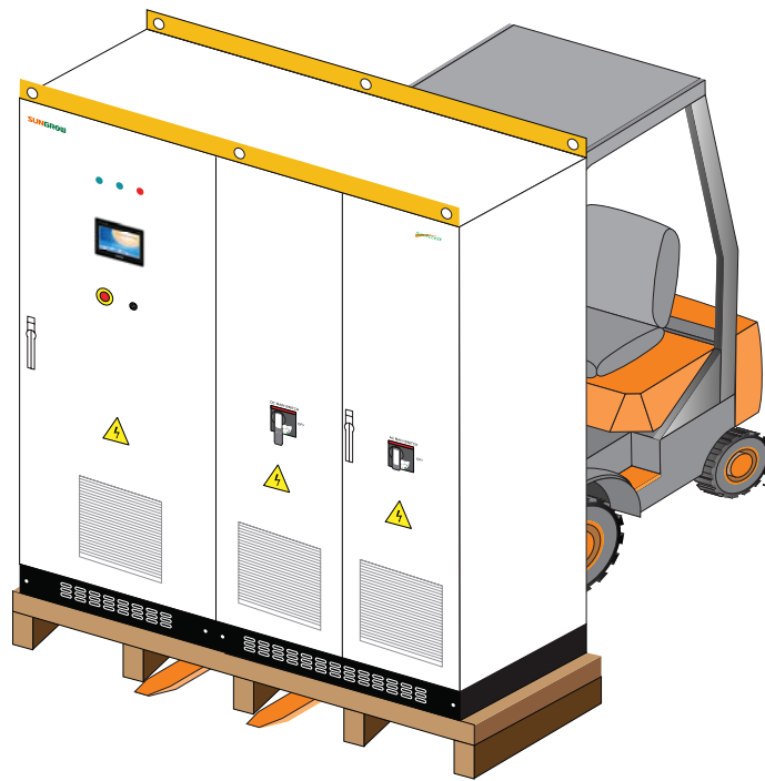
图7-2 叉车运输
