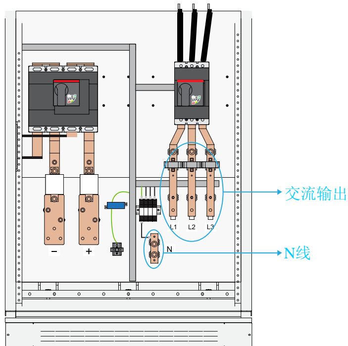
图8-7 交流侧接线端子
