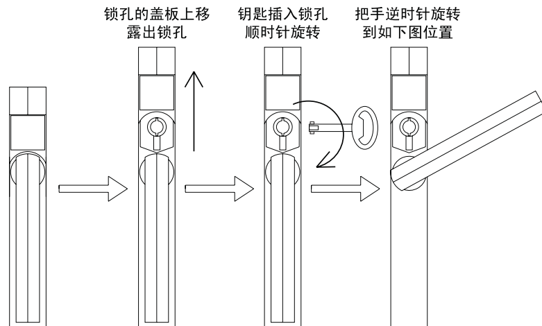
图8-3 开启前门
