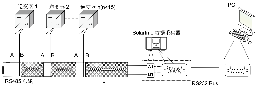
图8-12 数据采集器和 PC 机通过 RS485 进行监控
