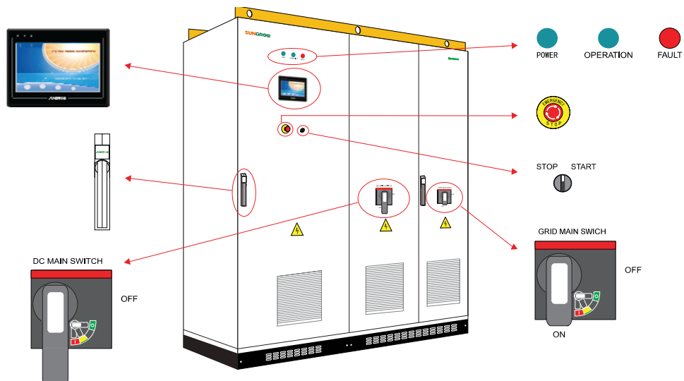
图4-4 SG250K3 外观图
