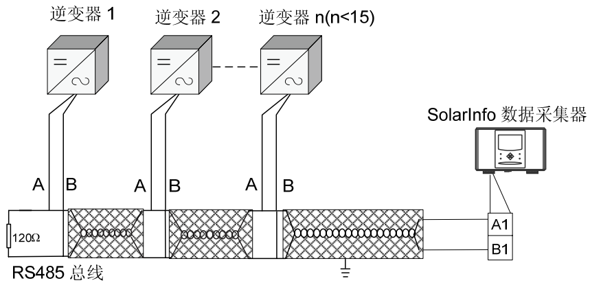
图8-10 数据采集器通过 RS485 进行监控
