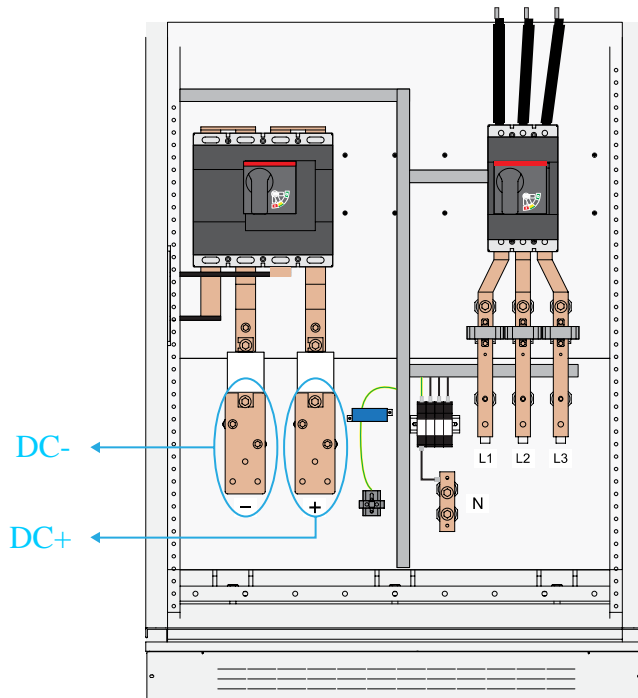
图8-5 直流侧接线端子
