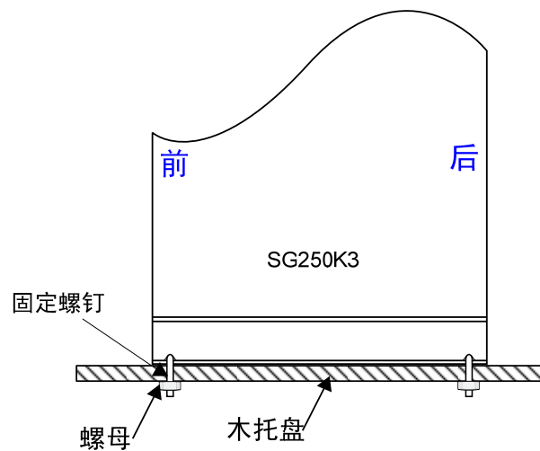
图7-5 固定在木托盘上
