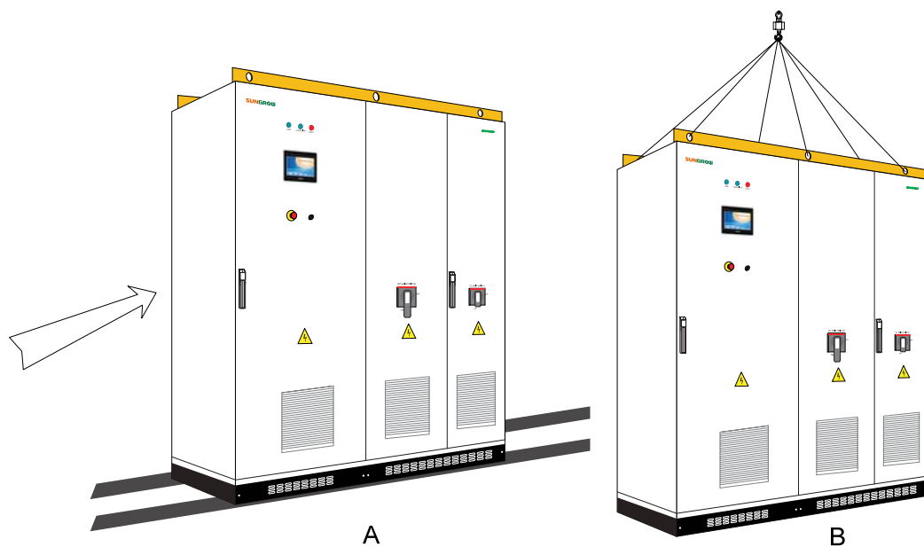
图7-4 滑动或起吊方式移动逆变器
