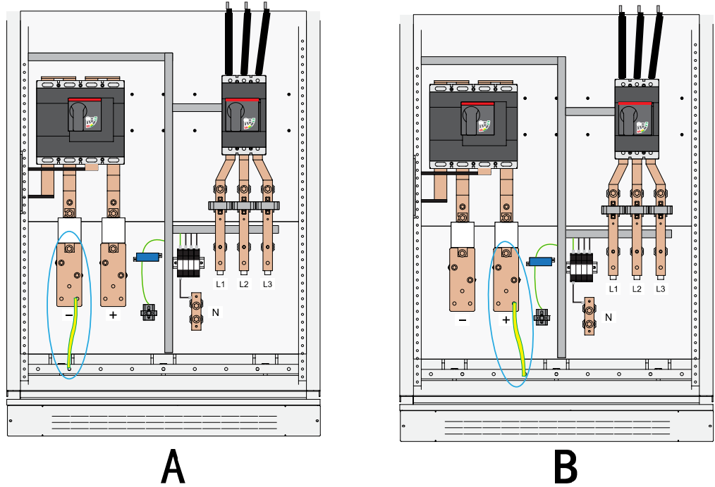
图8-6 直流输入接地连接
