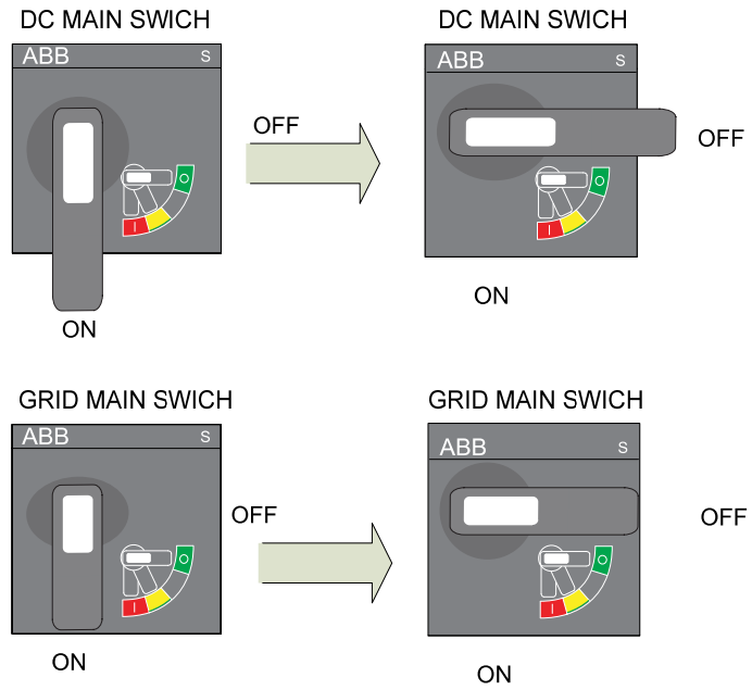
图8-2 关闭断路器
