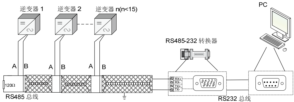
图8-11 PC 机通过 RS485 进行监控
