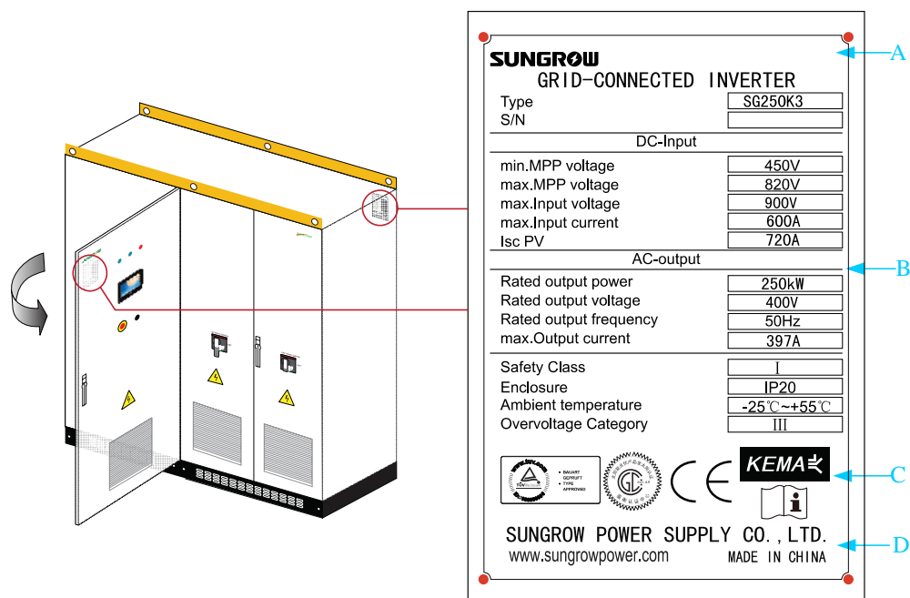
图3-1 SG250K3 铭牌及位置示意（图片仅供参考，请以实物为准）
