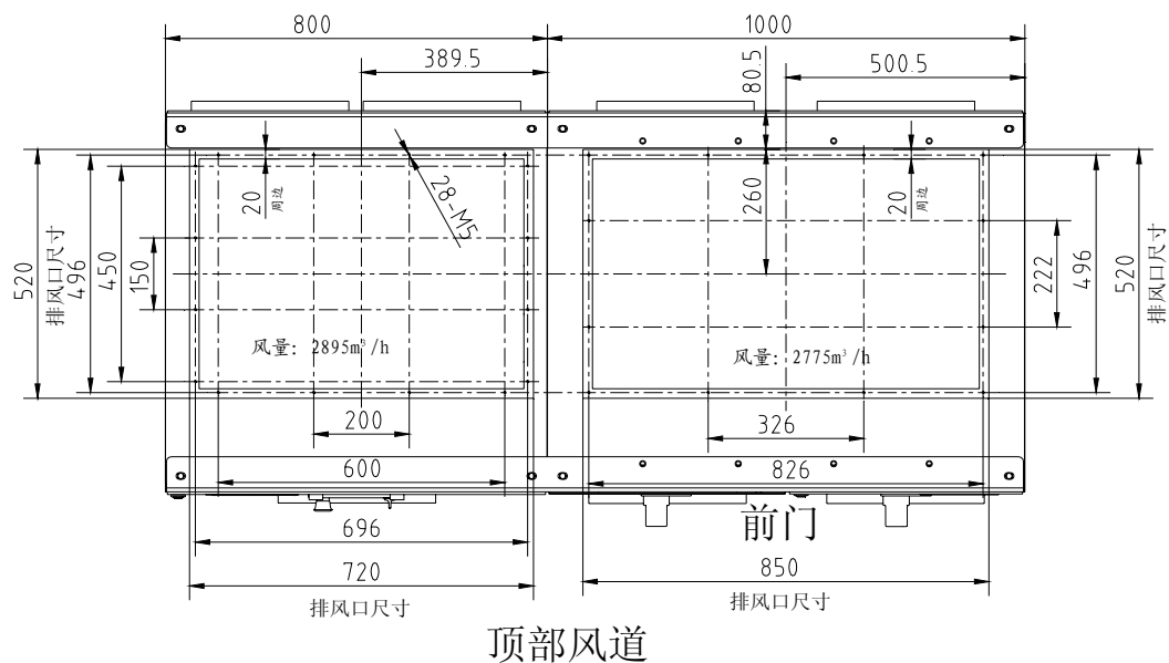
图4-3 顶部出风口
