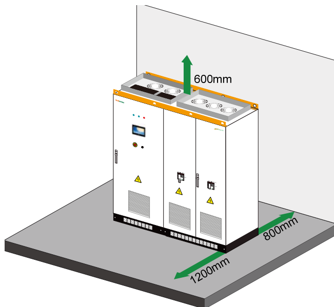
图5-2 SG250K3 安装空间距离
