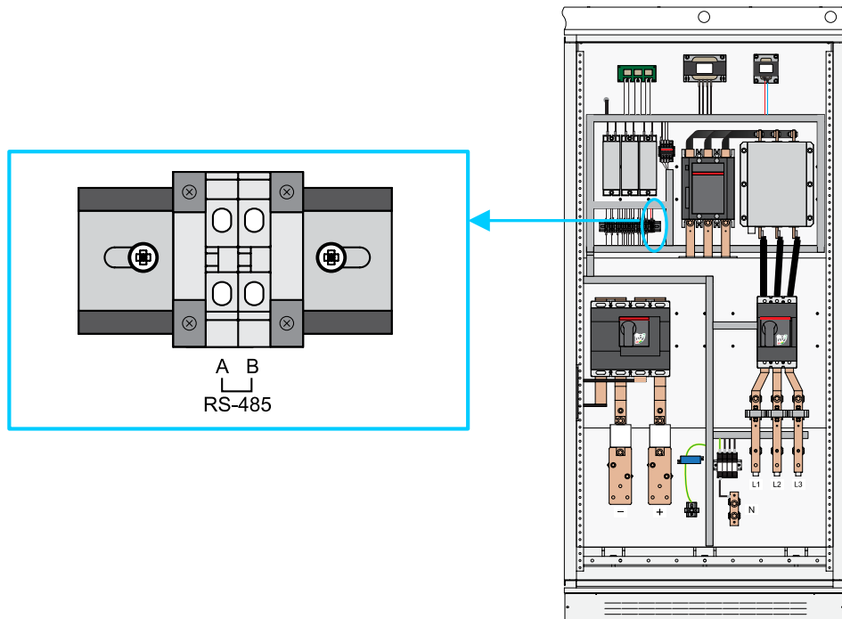
图8-9 通讯系统接线图
