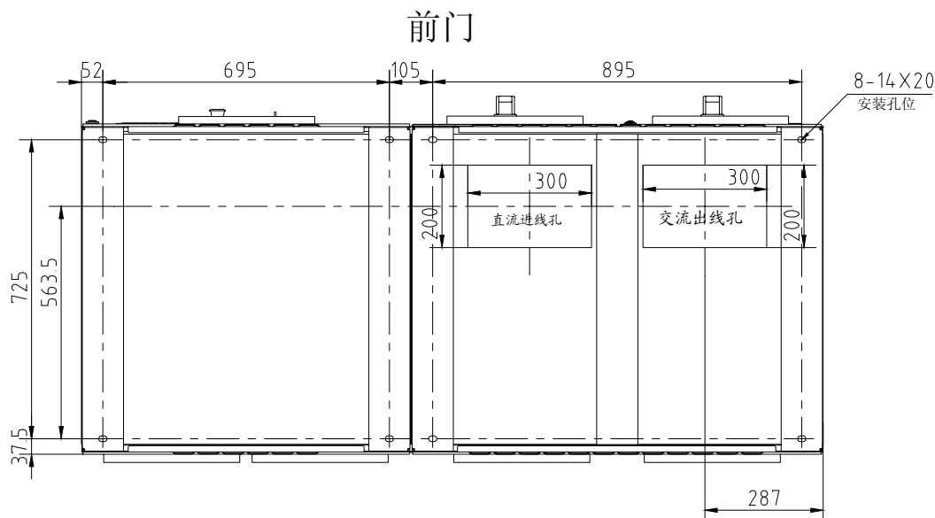
图4-2 SG250K3 底部视图
