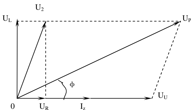
图 3 光伏发电并网运行的电路矢量图
