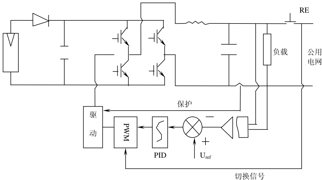
图 5 市电断电时单独运行方式
