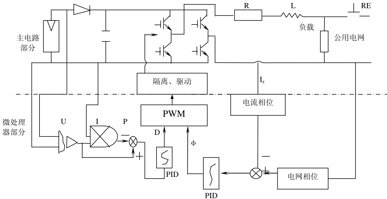
图 4 光伏发电并网运行专用逆变器的结构
