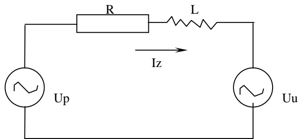
图 2 光伏发电并网运行的电路原理图
