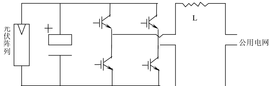
图 1 光伏发电并网原理
